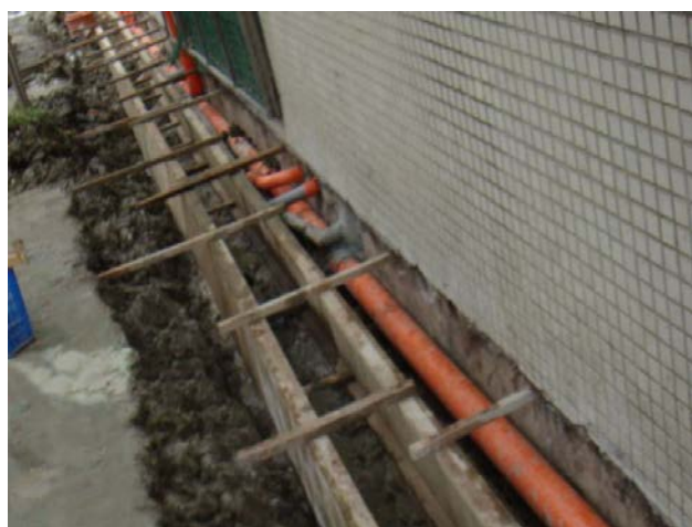
臺北市污水下水道用戶接管施工照片 (臺北市政府工務局衛生下水道工程處提供)
