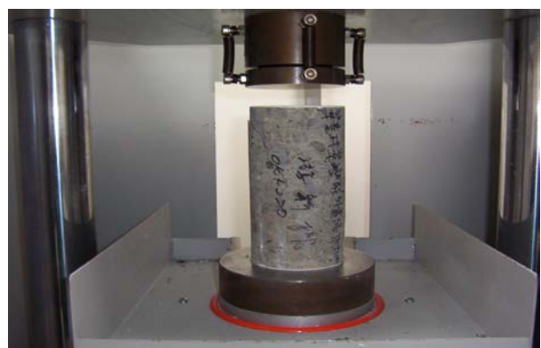
混凝土鑽心試體試驗情形 (南投縣政府提供)
